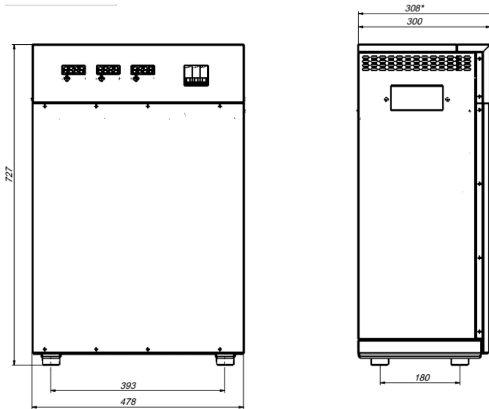
Рисунок 4. Габаритні розміри стабілізаторів Мережик Х-3х5.5/7/9/11/14
