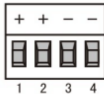
Рисунок 11: Порт RS485
